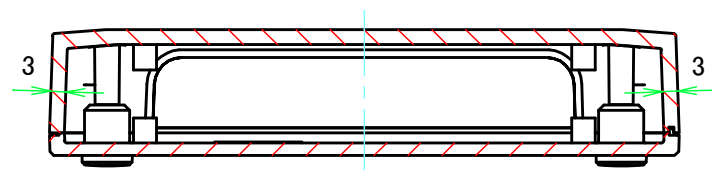
B-B ( 1 : 1.5 )
