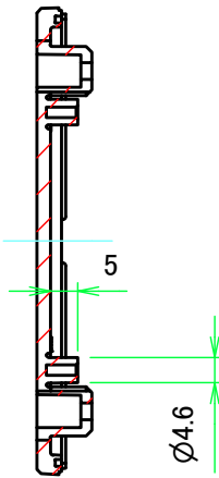
E-E ( 1 : 1.5 )
